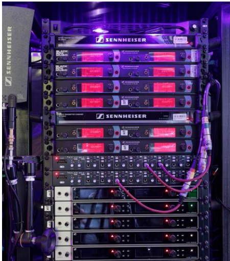
Monitorsender der Serie 2000 IEM und Mikrofonempfänger der Serie Digital 6000 von Sennheiser
